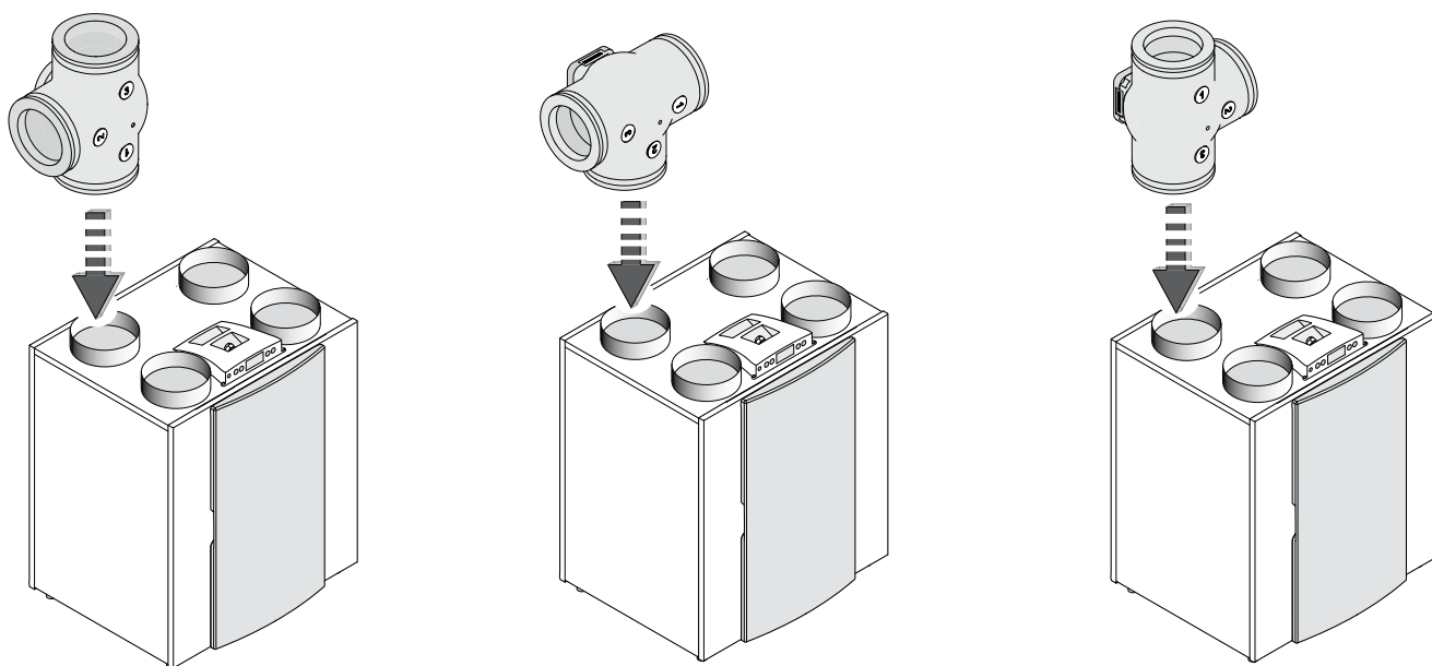
Anschlussbeispiele eines Zonenventils an den Zuluftkanal des WRG-Geräts
