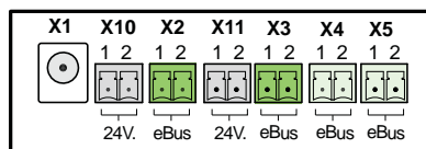
Anschlüsse am Zonenventil
