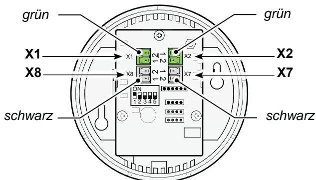
Anschlüsse am CO 2 -Sensor
